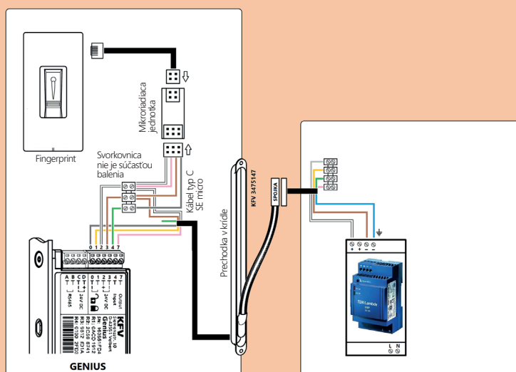
Krídlo dverí
