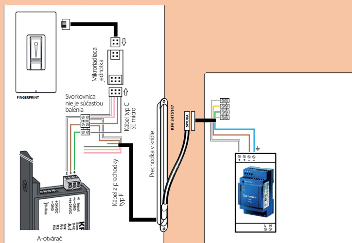
Krídlo dverí
