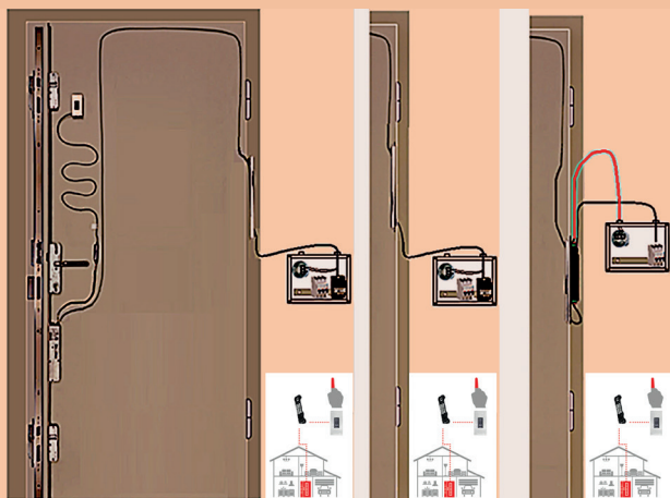
Prechodka v zárubni
