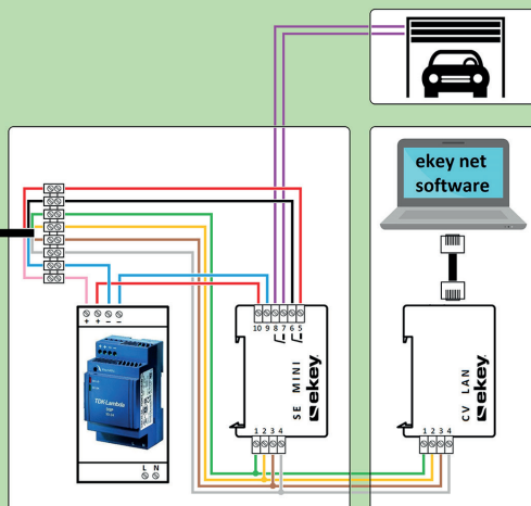
Elektrický rozvádzač
