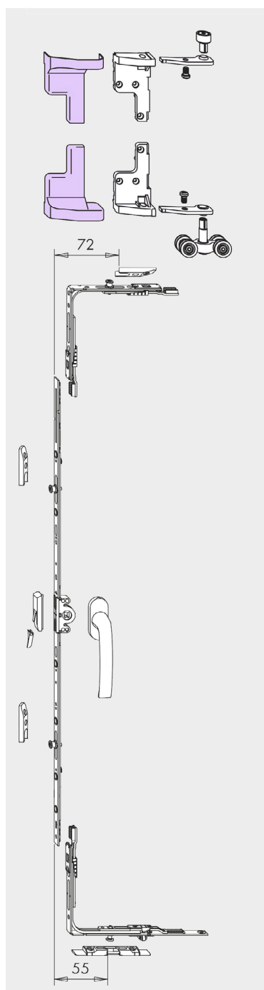
SPOJ „D“
