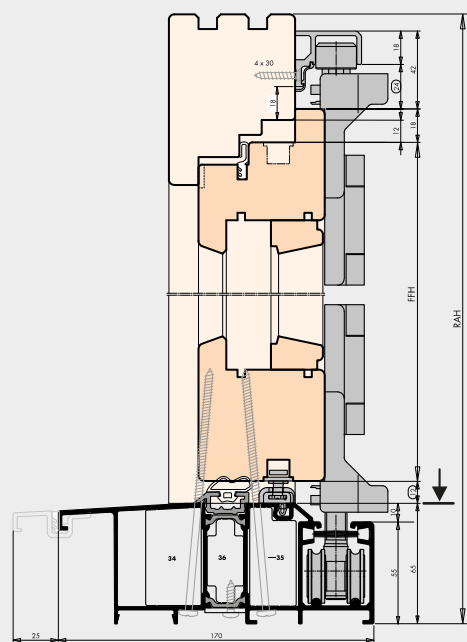
Dnu otvárajú portál, dole s bezbariérovým profilom
