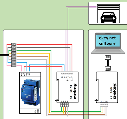
Elektrický rozvádzač
