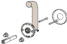
ROZPERNÝ ŠTVORHRAN EFHA SO ZAIŠŤOVACOU HLAVOU paniková garnitúra-kľučka / slepá montáž
