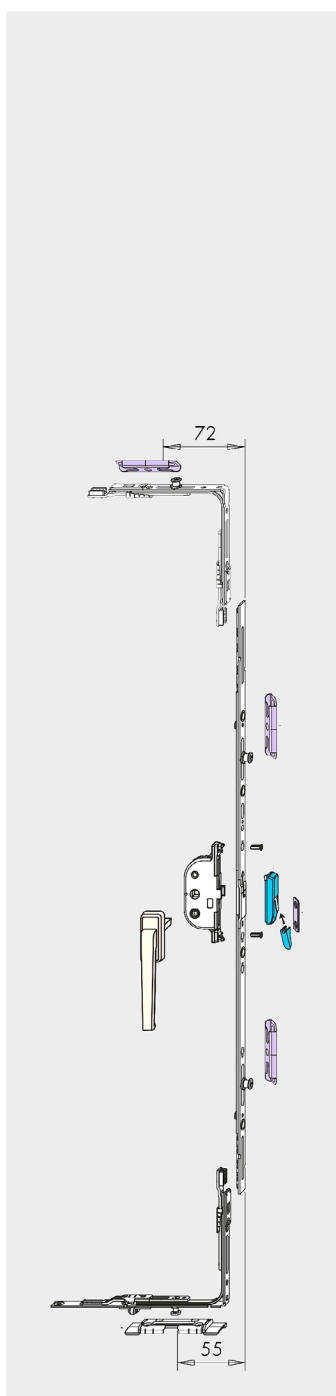
SPOJ „E“
