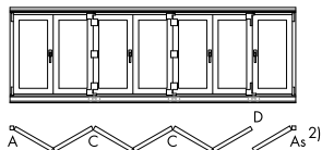
Schéma 761
