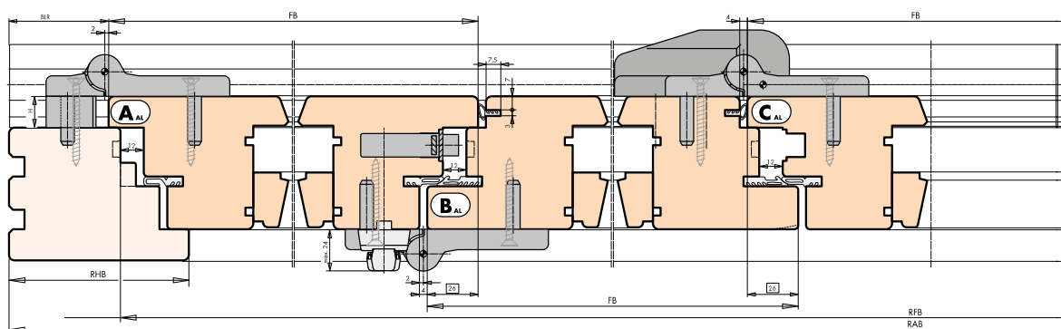
SPOJ „B“
