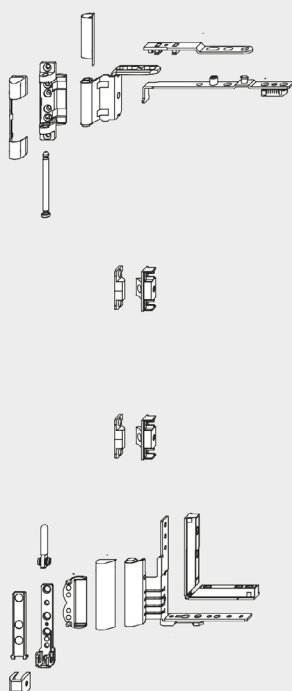
SPOJ „A“
