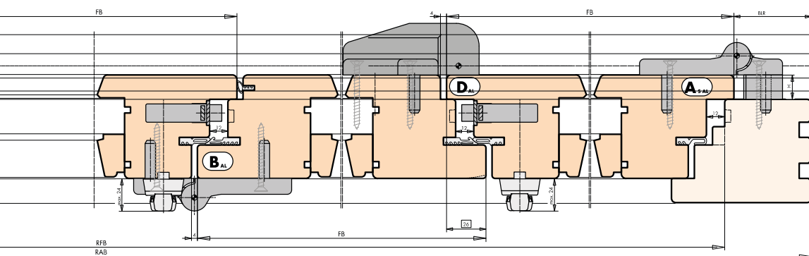
SPOJ „D“
