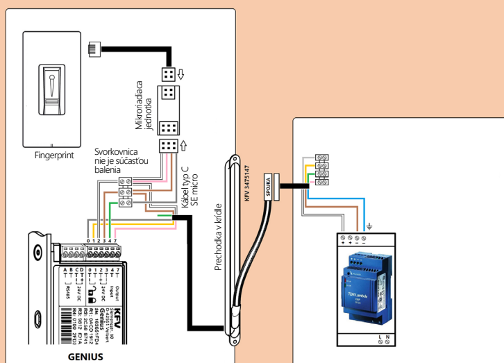
Křídlo dveří
