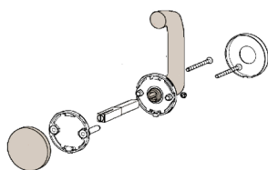
ROZPERNÝ ŠTVORHRAN EFHA SO ZAIŠŤOVACOU HLAVOU + redukcia paniková garnitúra-kľučka / záslepka
