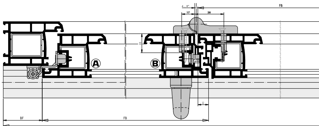
SPOJ „B“
