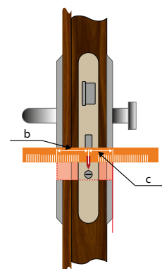
Falcové dvere
