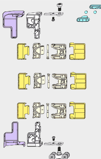
SPOJ „C“
