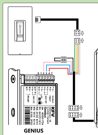
Krídlo dverí
