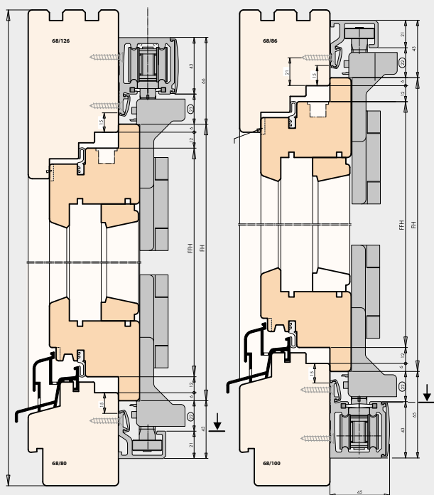
Dnu otvárajú portál, dole s priznaným rámom
