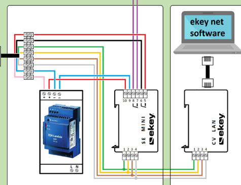
Elektrický rozvádzač
