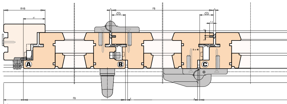
SPOJ „B“
