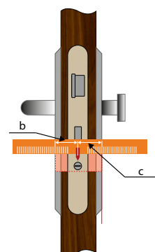
Bezfalcové dvere
