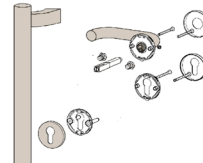
ROZPERNÝ ŠTVORHRAN EFHA SO ZAIŠŤOVACOU HLAVOU paniková garnitúra-kľučka / slepá montáž
