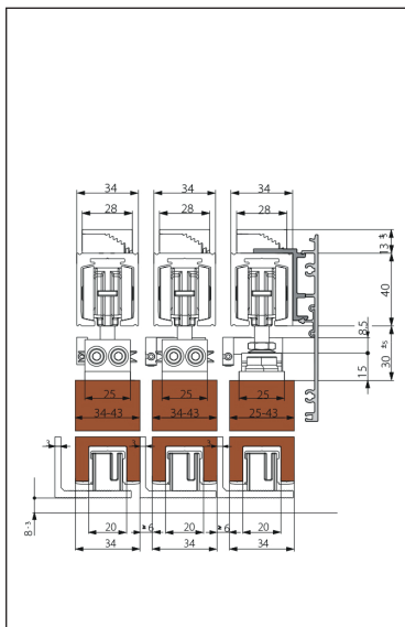
Montáž do stropu, spodné vedenie do steny
