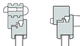
Montáž v ráme a v krídle
