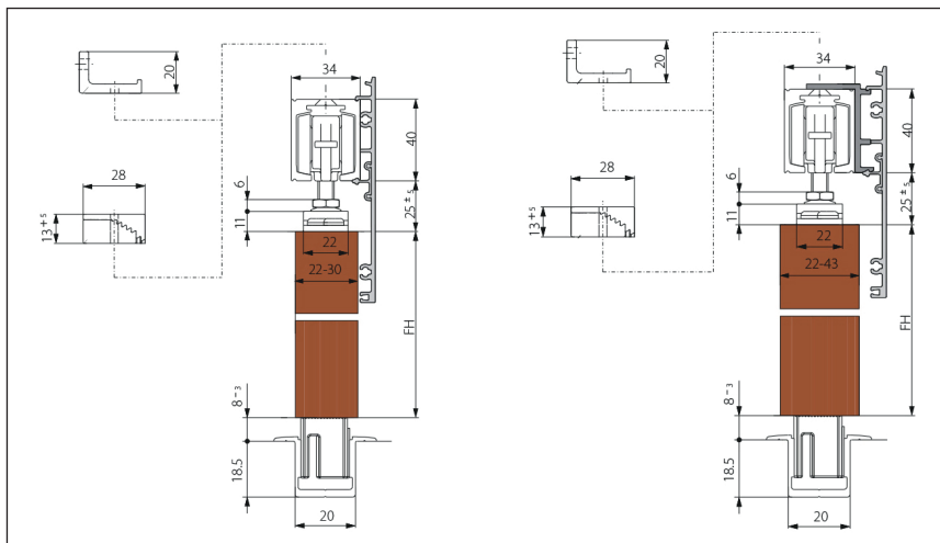
Montáž do stropu alebo do steny, spodné vedenie do podlahy
