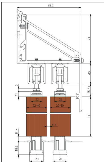
Montáž do steny, spodné vedenie do podlahy (systémové riešenie nie je sklado - objednávka podľa projektu)
