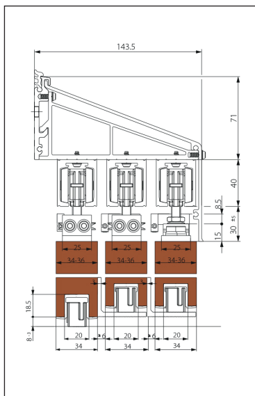
Montáž do steny, spodné vedenie do steny (systémové riešenie nie je sklado - objednávka podľa projektu)
